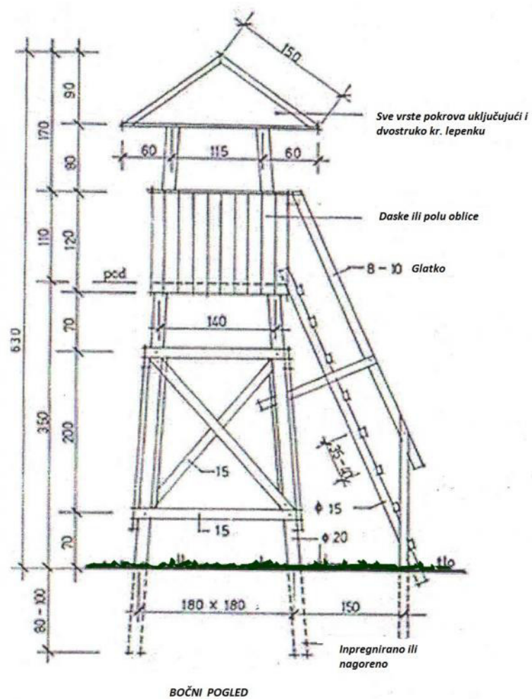
BOČNI POGLED
