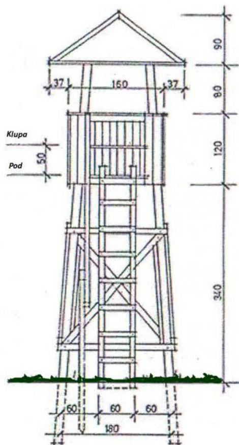
PREDNI POGLED
